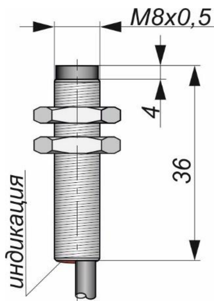
Габаритный чертеж
